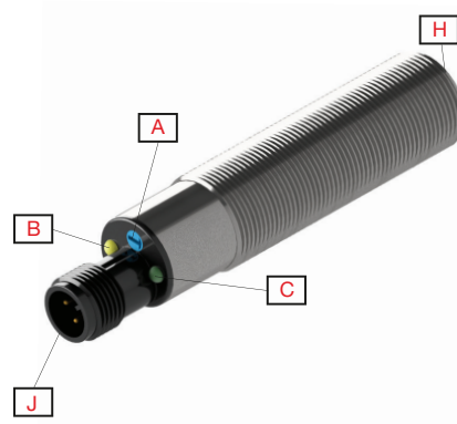
Fig. 2 CA18 Conducteur
